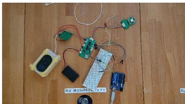
作成した試作用基板の写真
